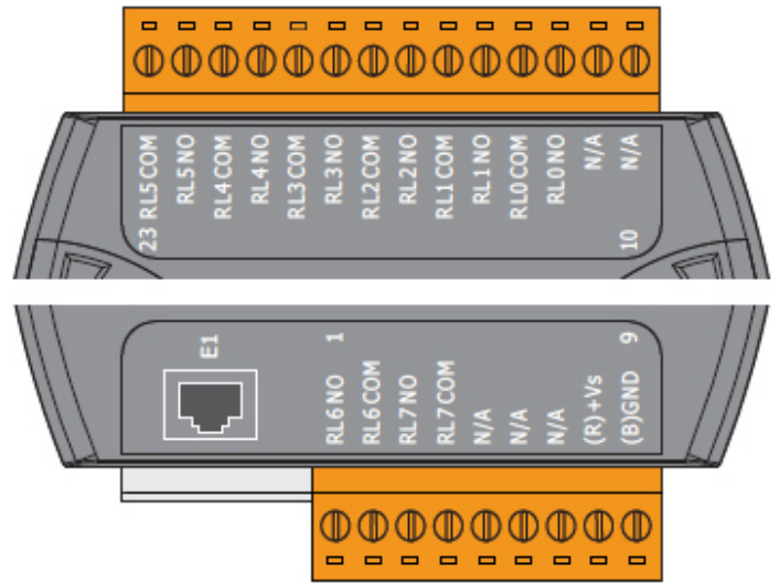
ETS-7267/PETS-7267
