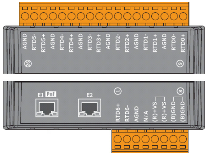
ETS-7215/PETS-7215
